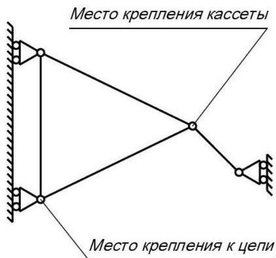
Рисунок 9 – Характерная кинематическая схема балансиров кассет
