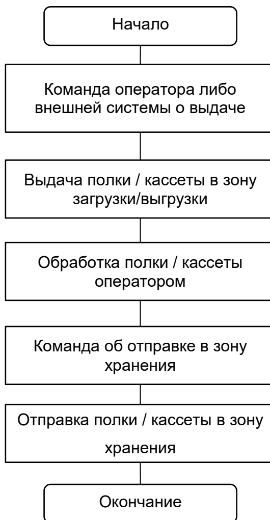
Рисунок 2 – Характерный цикл выдачи полки / кассеты
