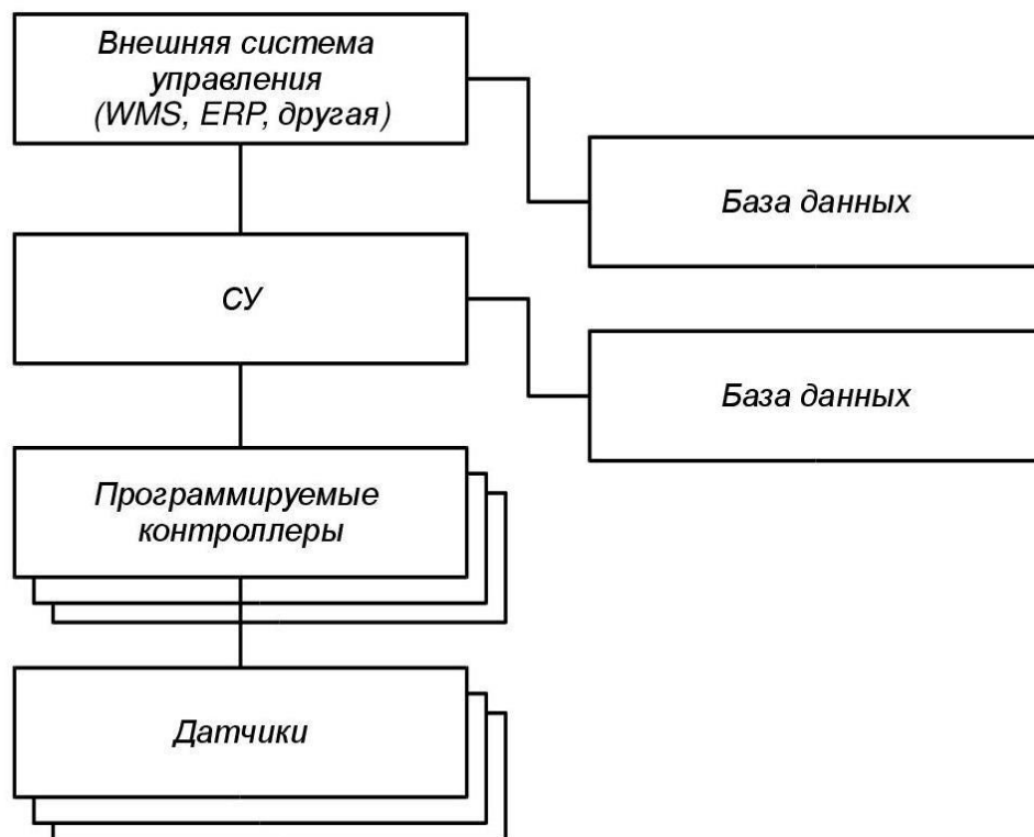
Рисунок 10 – Структурная схема управления лифтовой / элеваторной системой.
