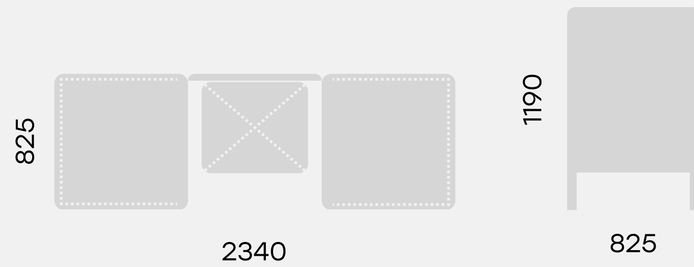
73.0138 Кабина 2-местная со столиком NAURA
