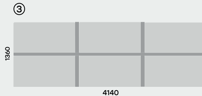
71.1023.140.70 Бенч-система D.SYS BC2-140x70-01
