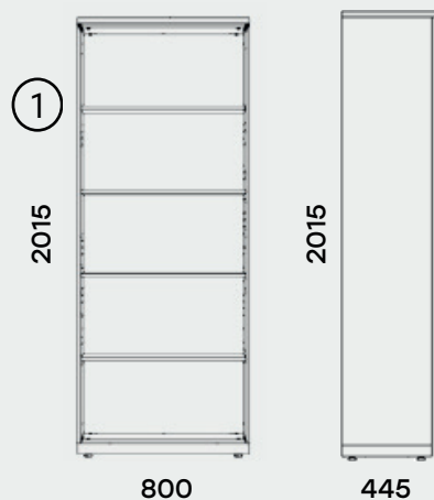
72.1001.80.5 Шкаф архивный большой OASYS ША-80x5-01
