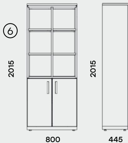
72.1006.80.5 Шкаф архивный большой OASYS ША-80x5-06
